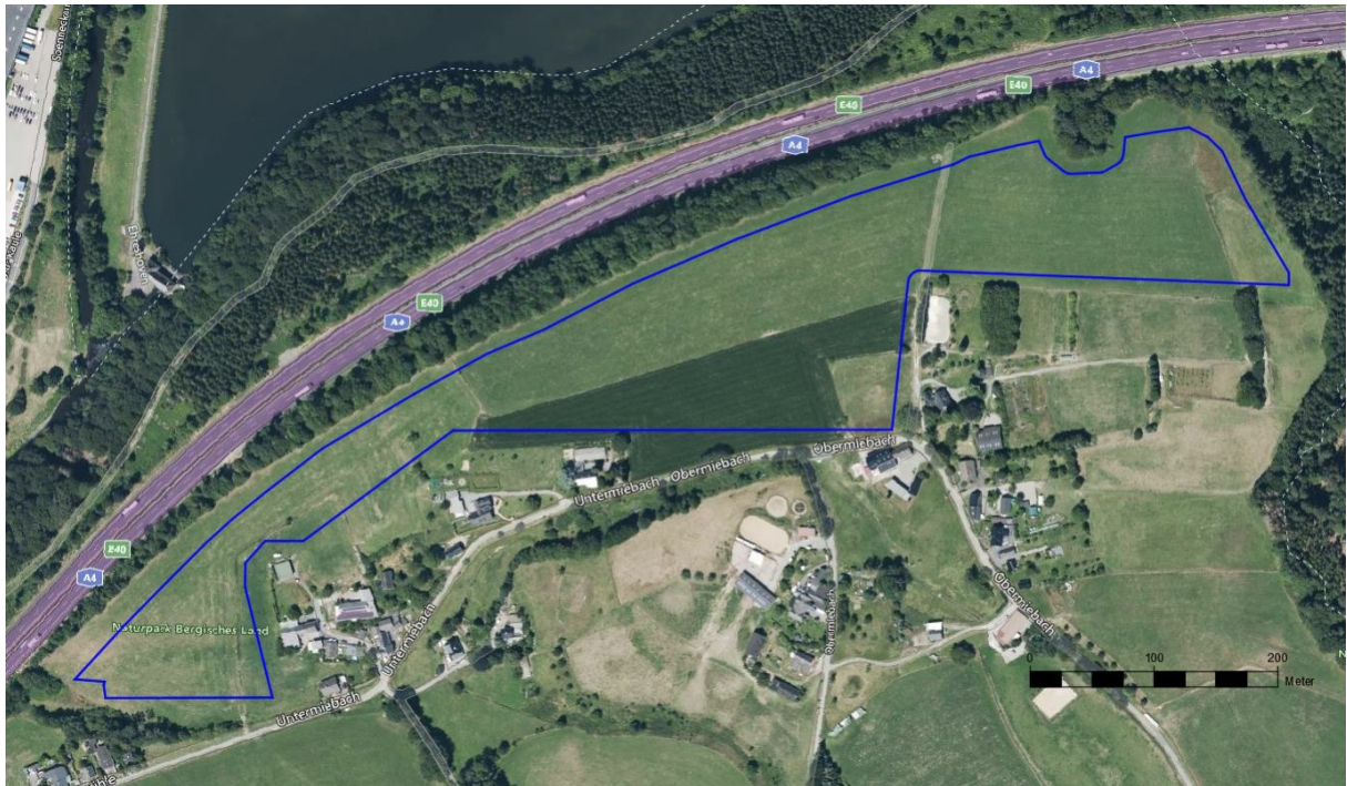
Geltungsbereich des Bebauungsplanes Nr. 162 PV-Freiflächenanlage „Obermiebach“ sowie der 83. Änderung des Flächennutzungsplanes PV-Freiflächenanlage „Obermiebach“.
