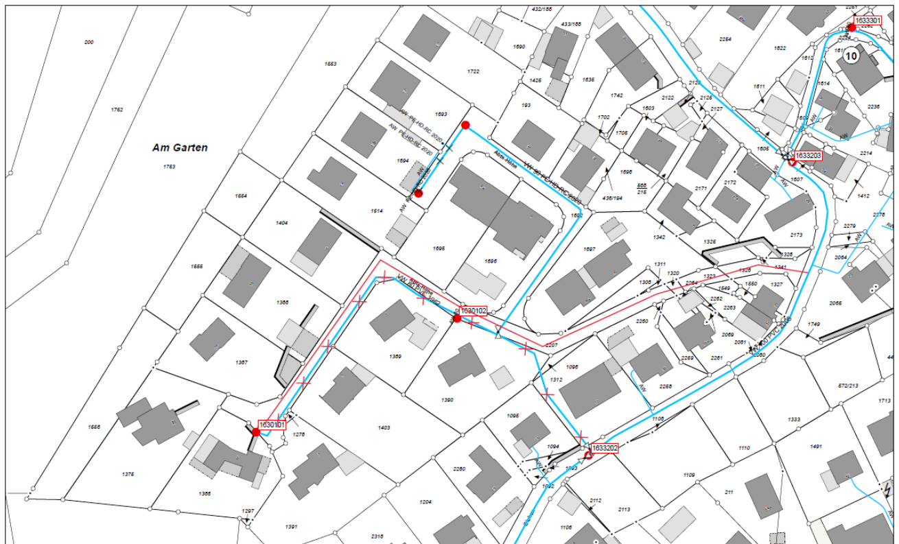
Abb. 1: Sanierungsbereich Abts-Höhe
